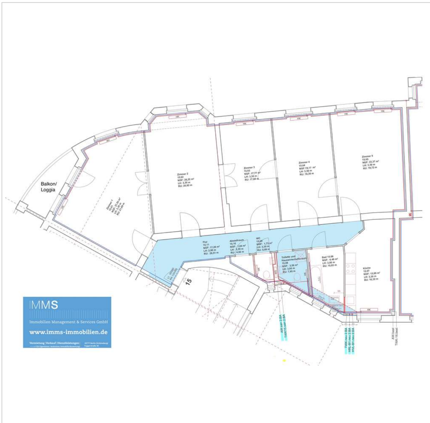
Obj.-Nr. 24240901 - Grundriss
