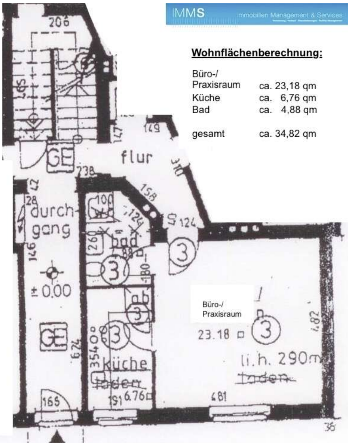
Obj.-Nr. 12241010 - Grundriss
