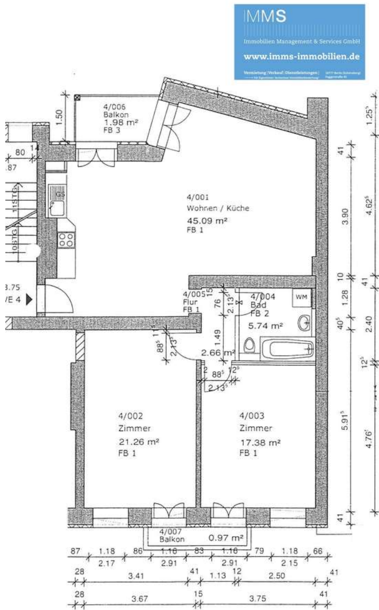
Grundriss 1.Obergeschoss
