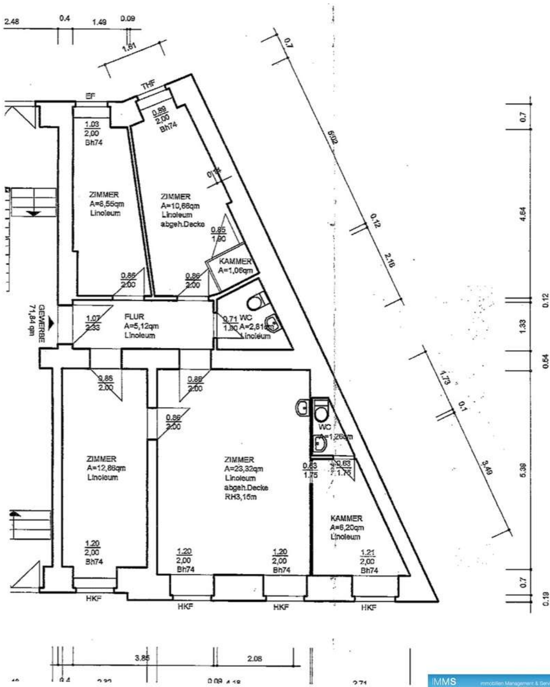
Obj.-Nr. 04190101 - Grundriss
