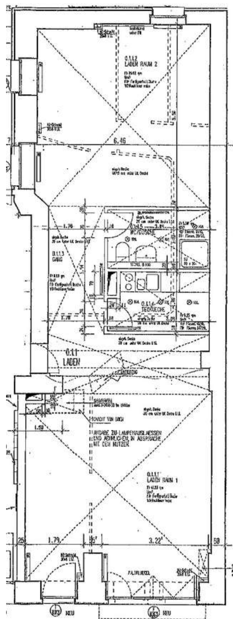
Obj.-Nr. 04250107 - Grundriss
